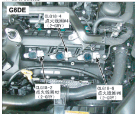
40. 发动机顶部
