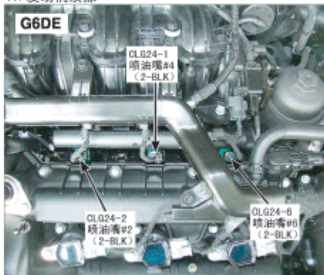
41. 发动机顶部
